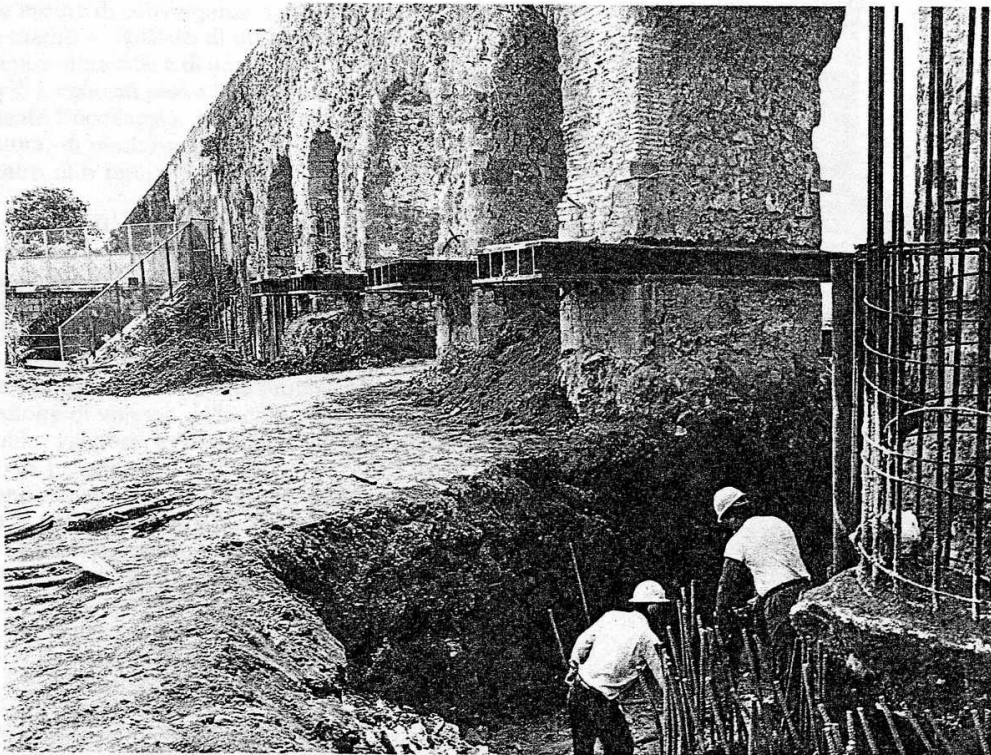
Fase di realizzazione di una spalla del sottopasso. Sullo sfondo a sinistra, l'imbocco lato Roma della galleria artificiale sotto l'Acquedotto della coppia di binari esistente della Roma-Cassino.
